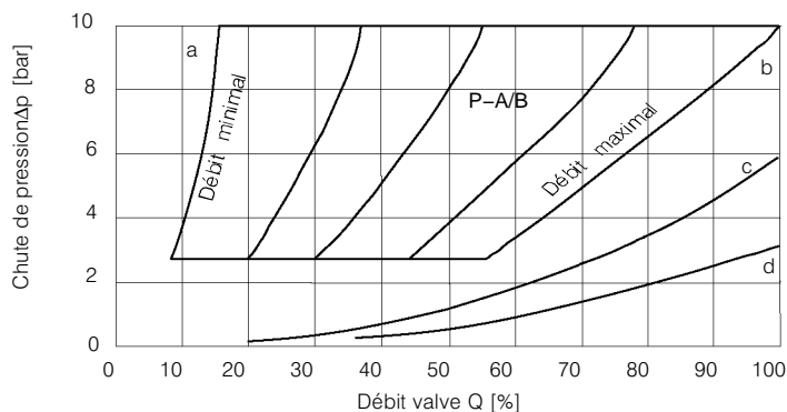
1.2.2 Figure: Chute de pression sur les arêtes de commande du tiroir principal en fonction du débit de la valve; cf. aussi tableau 1.2.1, page 4
