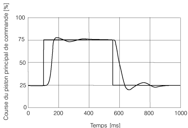
Fonction de passage pour signal électrique d'entrée échelonné 50 % ± 25 %.
