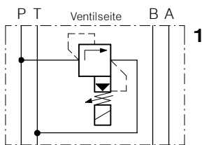
SWUVPZ-1...-PT-FB-6 ... SWUVPZ-1...-PT-FB-6 ...
